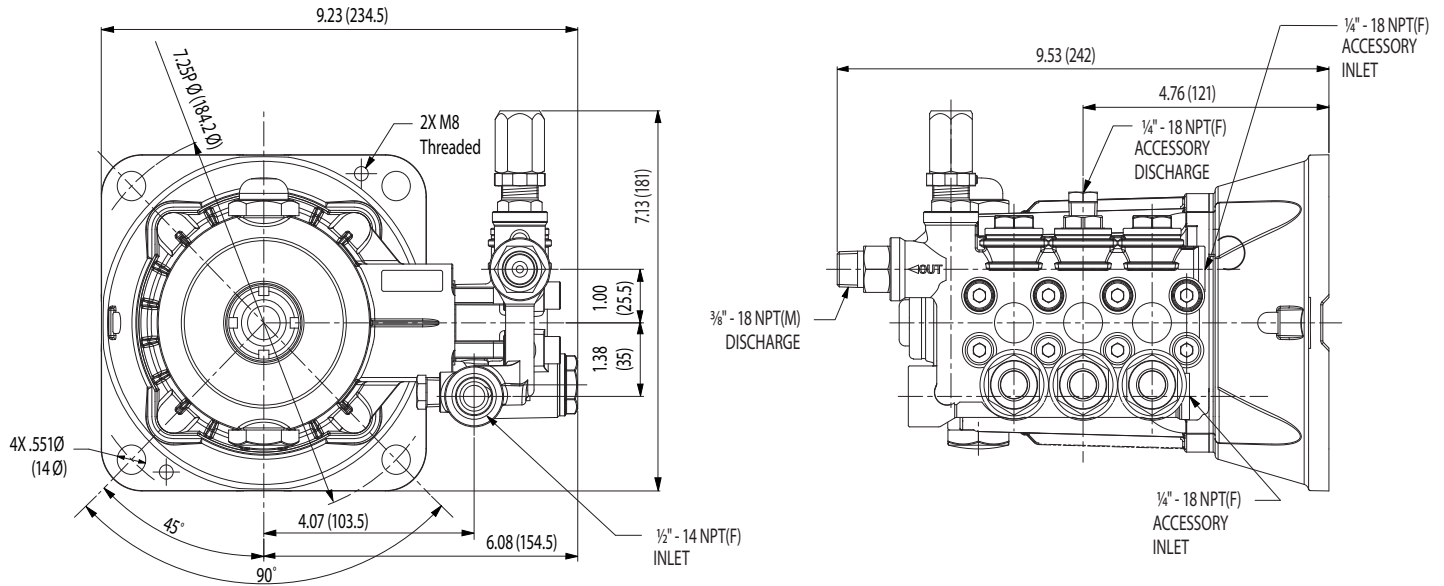
Base Models 5SP30ELR, 5SP35ELR, 5SP40ELR
